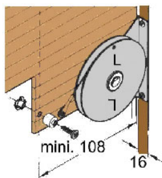
Dimensions de montage
