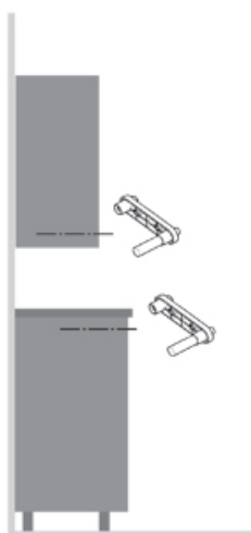
Maintien magnétique en position fermée (versions standard et design)
