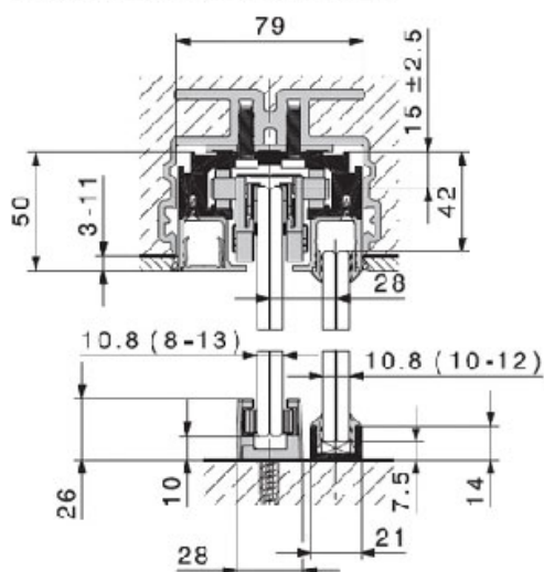
Intégration dans plafond en béton
