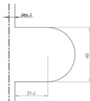
Porte encastrée
